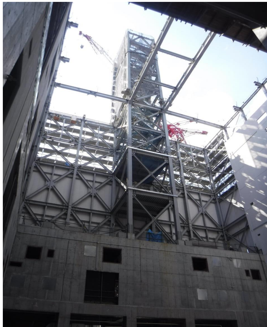
●1工区煙突鉄骨組立完了
