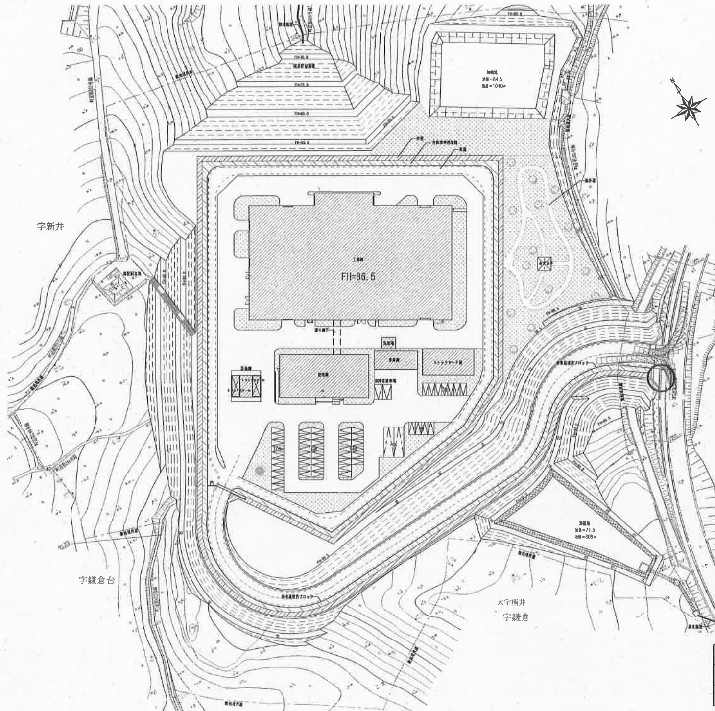
埼玉西部環境保全組合 次期更新施設基本計画 配置図 S=1/1000
